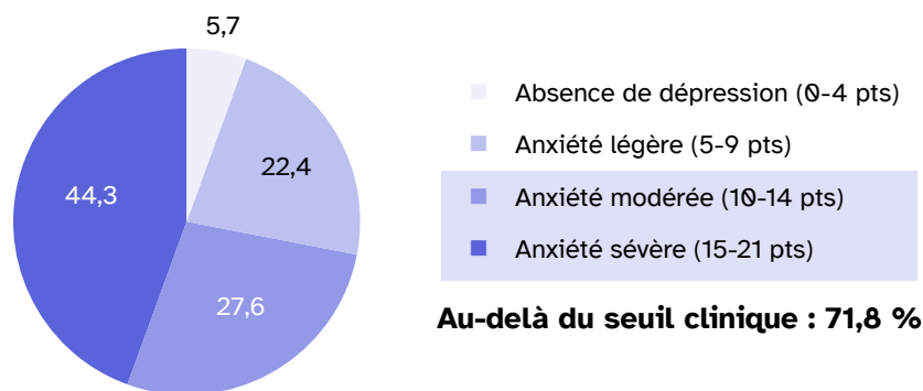
Figure 21 : Seuils cliniques d'anxiété
